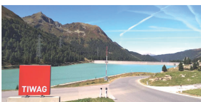
Längentaler Stausee
